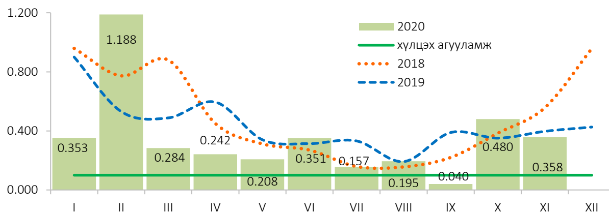
Зураг 10. Улаанбаатар 3 хотын агаар дахь 10 микроноос бага хэмжээтэй тоосны агууламж, 14 харуулын дундаж, сараар, мг/м 3
