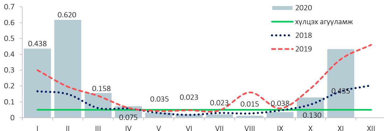
Зураг 7. Улаанбаатар 4 хотын агаар дахь хүхэрлэг хийн агууламж, 12 харуулын дундаж, сараар, мг/м 3
