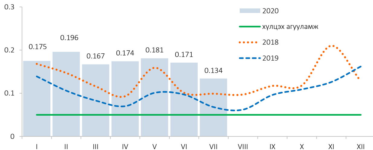
Зураг 8. Улаанбаатар 3 хотын агаар дахь азотын давхар ислийн агууламж, 15 харуулын дундаж, сараар, мг/м 3
