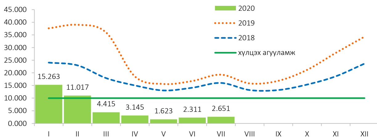
Зураг 9. Улаанбаатар 3 хотын агаар дахь нүүрстөрөгчийн дутуу исэл, 15 харуулын дундаж, сараар, мг/м 3
