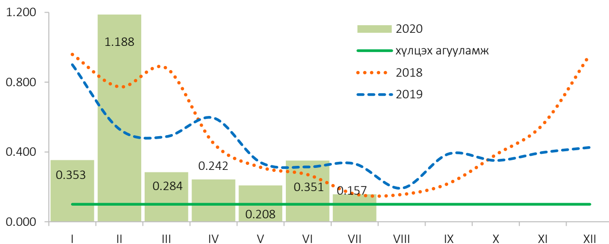
Зураг 10. Улаанбаатар 3 хотын агаар дахь 10 микроноос бага хэмжээтэй тоосны агууламж, 15 харуулын дундаж, сараар, мг/м 3
