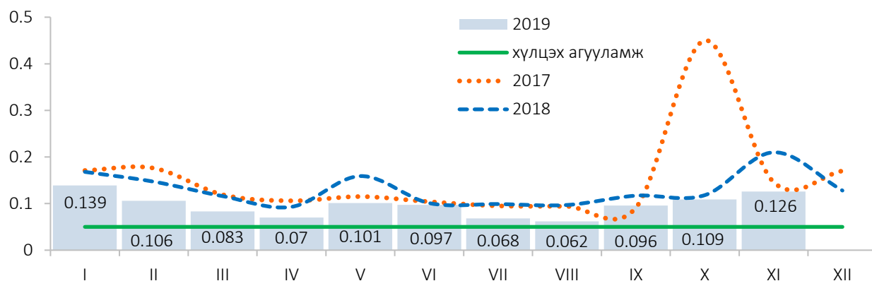
Зураг 10. Улаанбаатар 3 хотын агаар дахь нүүрстөрөгчийн дутуу исэл, 15 харуулын дундаж, сараар, мг/м 3
