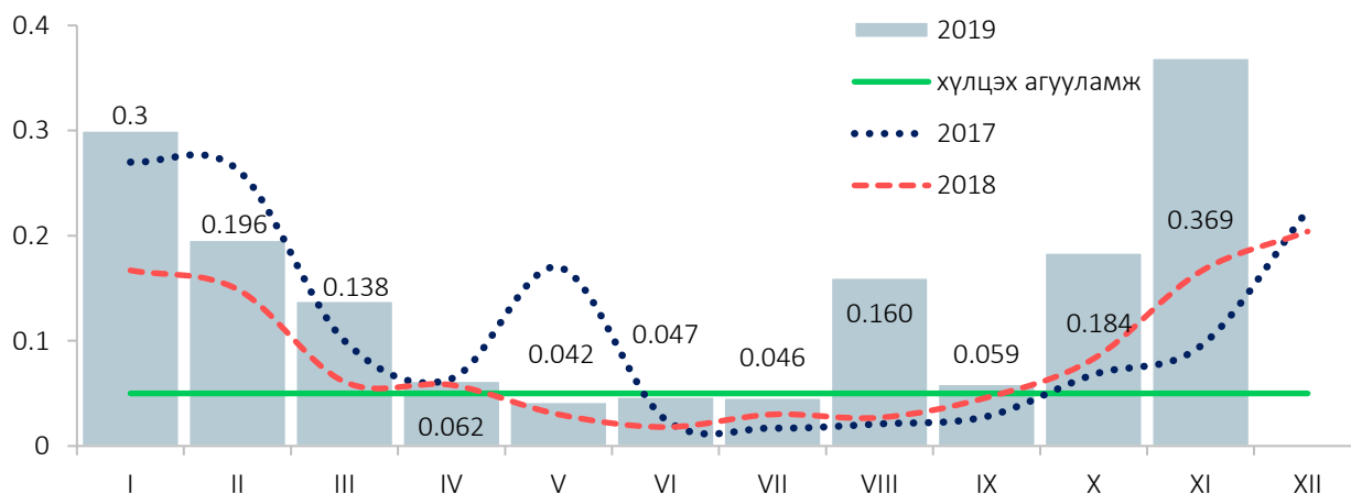
Зураг 8. Улаанбаатар 3 хотын агаар дахь хүхэрлэг хийн агууламж, 15 харуулын дундаж, сараар, \text{мг}/\text{м}^3
