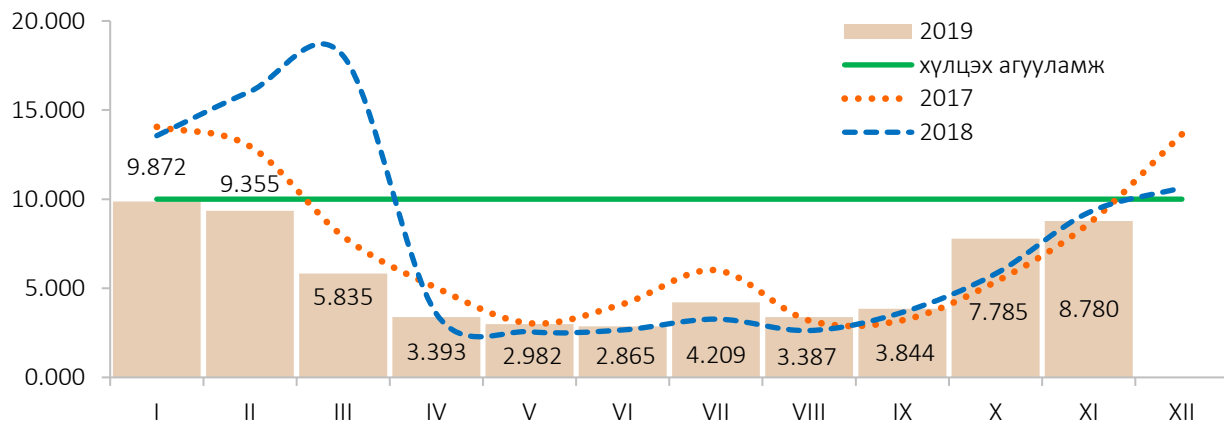
Зураг 11. Улаанбаатар 3 хотын агаар дахь 10 микроноос бага хэмжээтэй тоосны агууламж, 15 харуулын дундаж, сараар, мг/м 3
