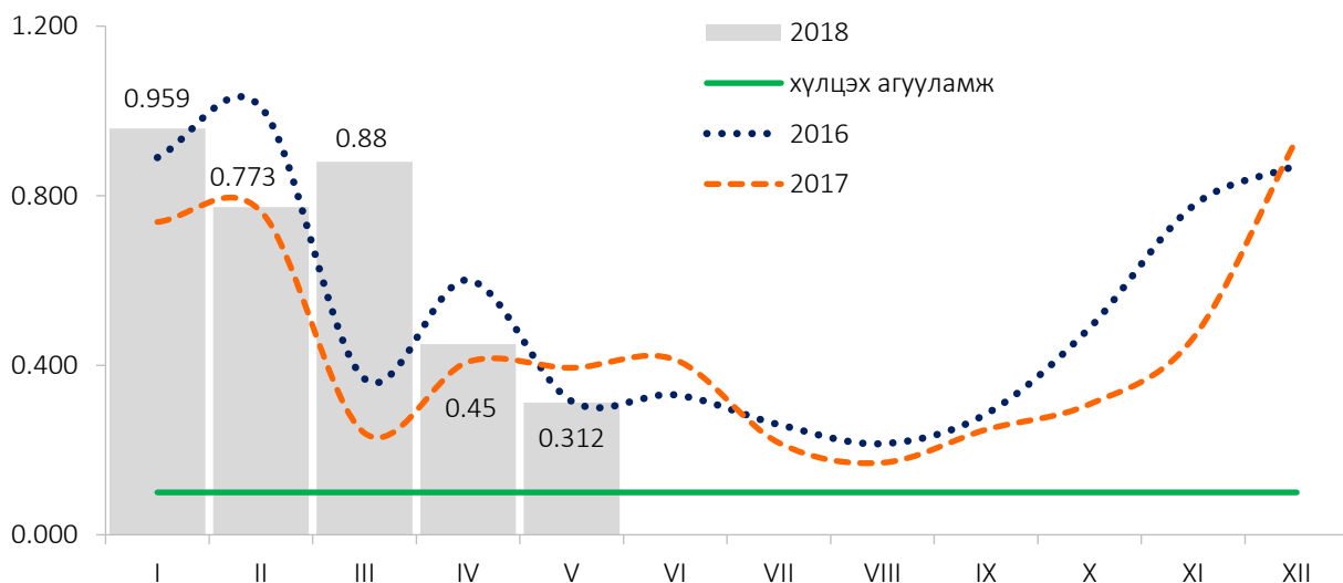
Зураг 9. Улаанбаатар 3 хотын агаар дахь 10 микроноос бага хэмжээтэй тоосны агууламж, 12 харуулын дундаж, сараар, мг/м 3
