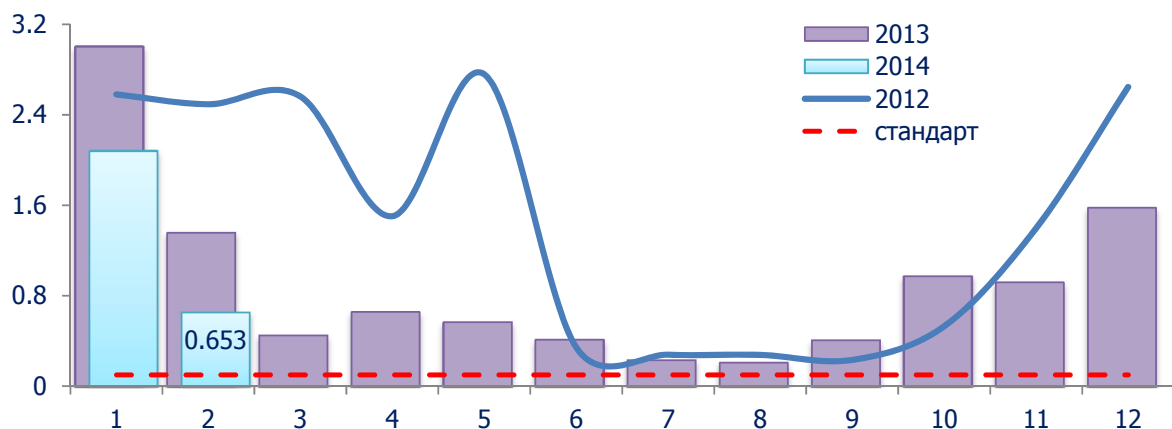
Зураг 28. Нүүрстөрөгчийн дутуу исэл, мг/м 3
