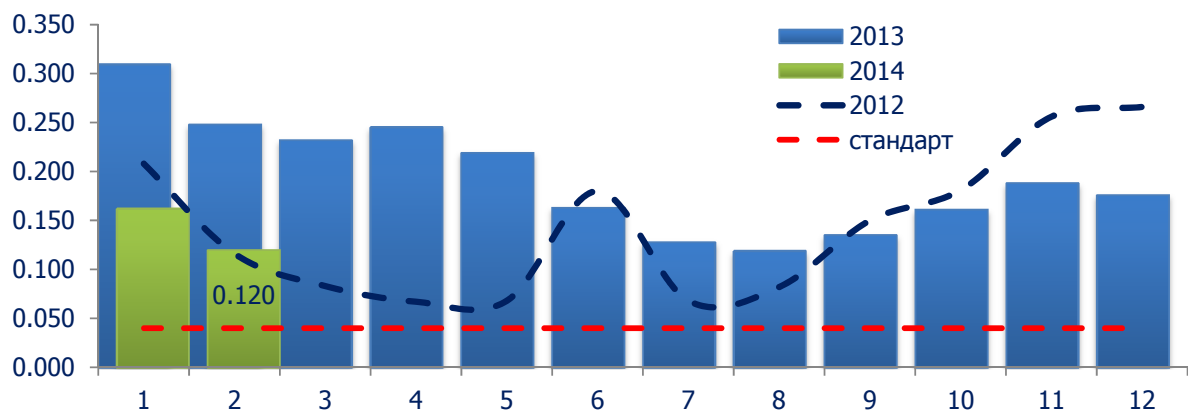
Зураг 26. Азотын давхар ислийн агууламж, мг/м 3
