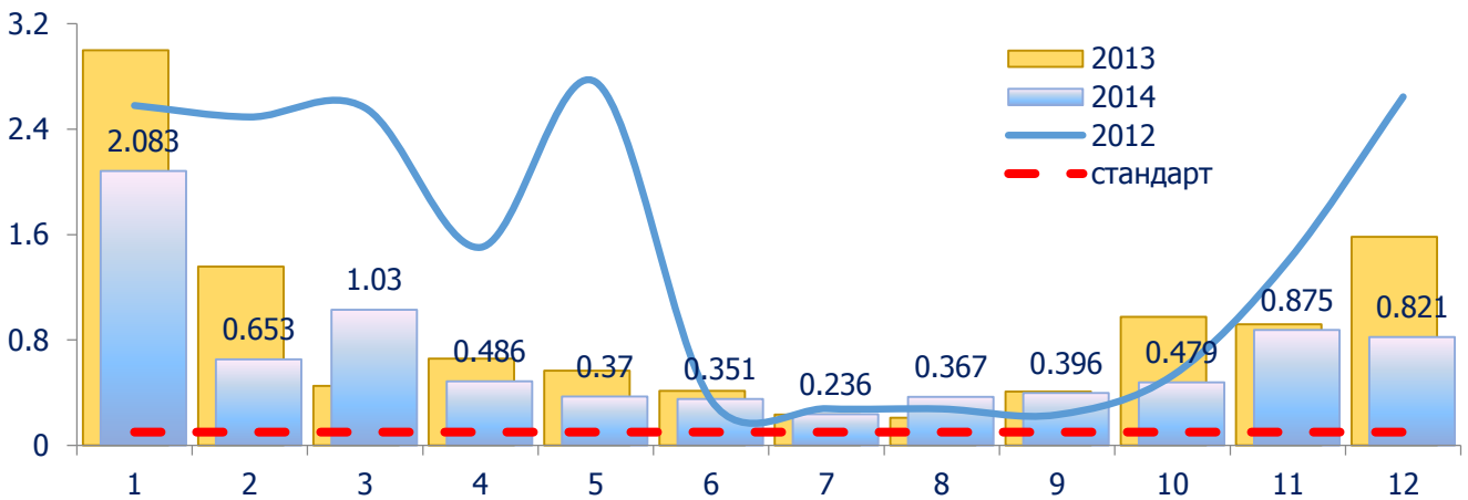
Зураг 45. Нүүрстөрөгчийн дутуу исэл, мг/м 3
