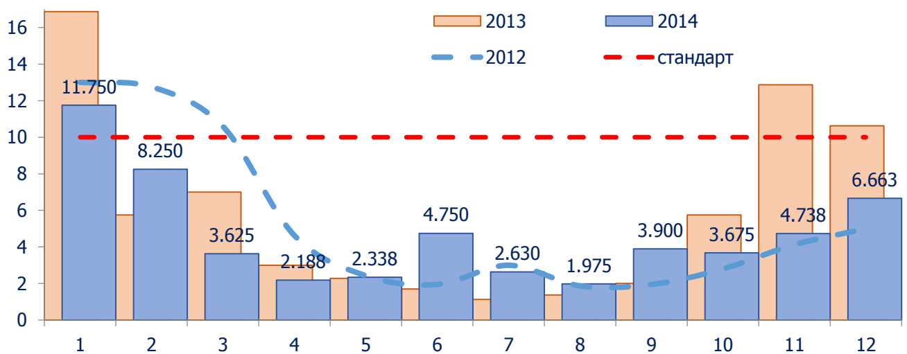
Зураг 45. Нүүрстөрөгчийн дутуу исэл, мг/м 3
